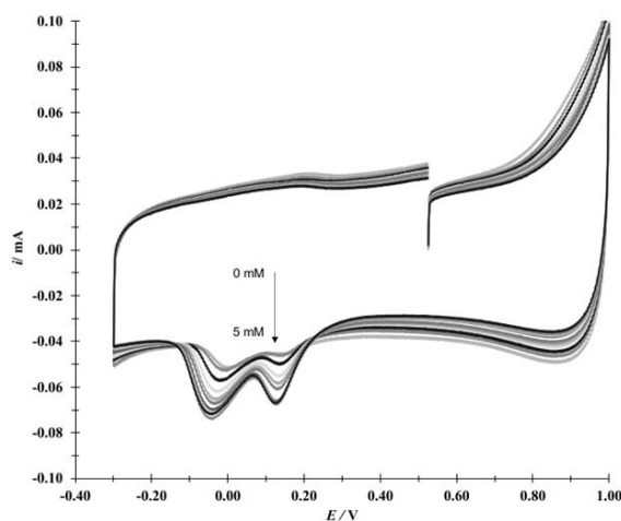
Figura 3. Familia de VC de Cr(III) sobre un EPC- \beta -CD vs Ag/AgCl, KCl sat a diferentes concentraciones de Cr(III) mostradas en la figura.
