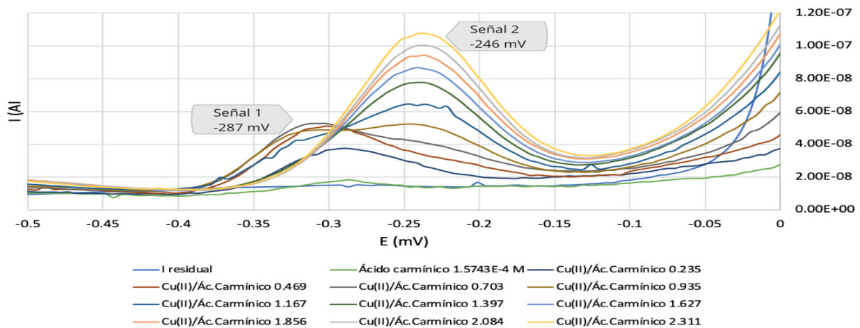
Figura 2. Polarograma diferencial de impulsos de ácido carmínico 1.5743 \times 10^{-4} \text{ mol L}^{-1} con diferentes concentraciones de Cu (II) y residual (blanco). Condiciones de trabajo: potencial de inicio 0 V, potencial final: -1.7 \text{ V} , velocidad de barrido: 0.005 \text{ V s}^{-1} , amplitud de impulso: 0.050 \text{ V} y tiempo de impulso: 0.040 \text{ s} . Medio: \text{NH}_4^+/\text{NH}_3 0.2 \text{ mol L}^{-1} a \text{pH}=10 .
