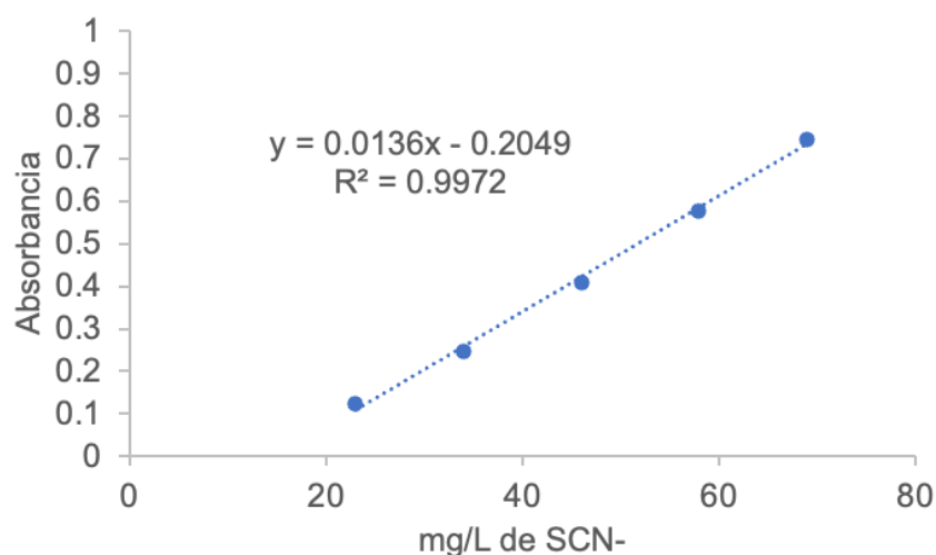
Figura 3. Ejemplo de curva de calibrado que se obtuvo para la cuantificación de \text{SCN}^- a 460 nm
