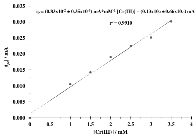
Figura 4. Gráfico |i_{pc}| = f([Cr(III)]) siguiendo el E_{pc} = 0.128 V en disolución amortiguadora a pH=5.
