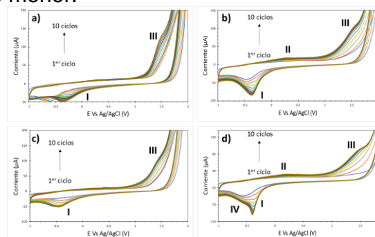
Figura 2. Voltamperogramas cíclicos de la electropolimerización de bCD sobre la superficie de un electrodo de carbón vitriro: a) pH 2, b) pH 3, c) pH 4 y d) pH 5.
