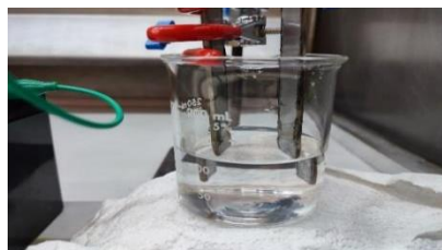
Figura 1. Celda electroquímica con muestra contaminada con hierro.
