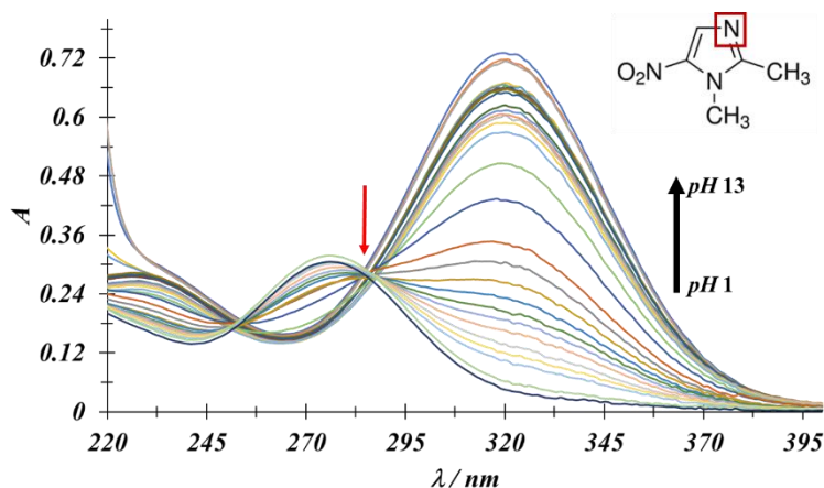
Figura 5. Familia de espectros de absorción de UV-Vis DMZ 90 \mu\text{M} a diferentes valores de pH mostrados en la figura. En el inserto se muestra la molécula de DMZ señalando el nitrógeno que se protonaría en la reacción ácido-base. La flecha de color rojo señala el punto isobéptico.
