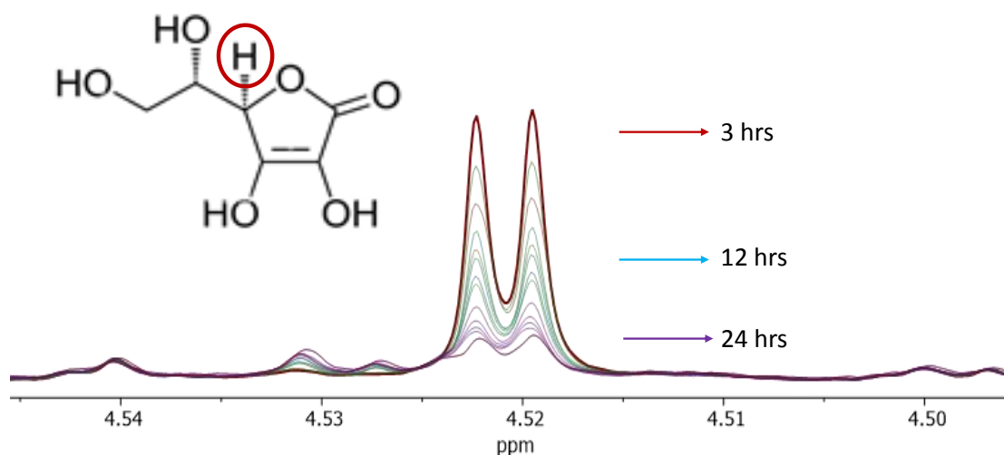
Figura 3. Ampliación de la región de los espectros de 1 H-RMN a 700 MHz de una muestra de jugo de limón a 27°C por 24 horas.
