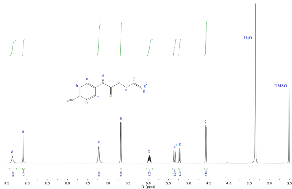
Figura 3. Espectro de RMN 1 H, (500 MHz, DMSO) del A4HPc.
