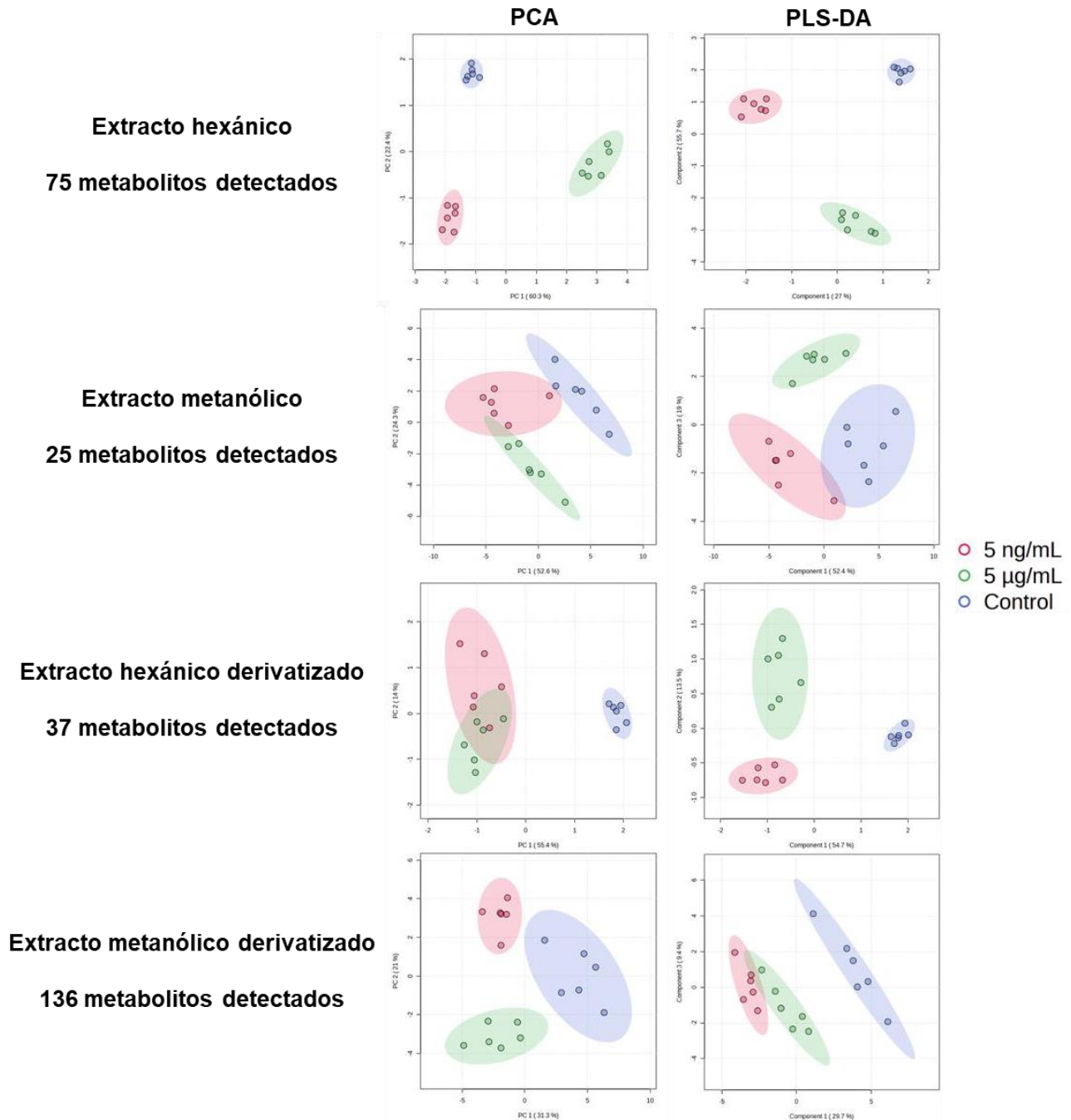
Figura 6. Gráficos de scores obtenidos del PCA y PLS-DA de la determinación del perfil metabólico de hojas de lechuga mediante UAE-GC-MS. Todos los análisis se realizaron calculando cinco componentes.
