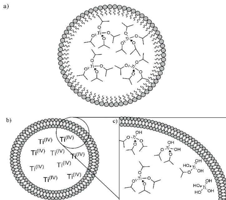
Figura 1 Esquema caricaturizado de 2 formas de interacción de agregados de DBSS con TIPT e intermediarios: a) modelo de micelas encerrando TIPT, b) modelo de vesículas encerrando especies de Ti(IV) c) acercamiento en el modelo de vesículas con posibles
