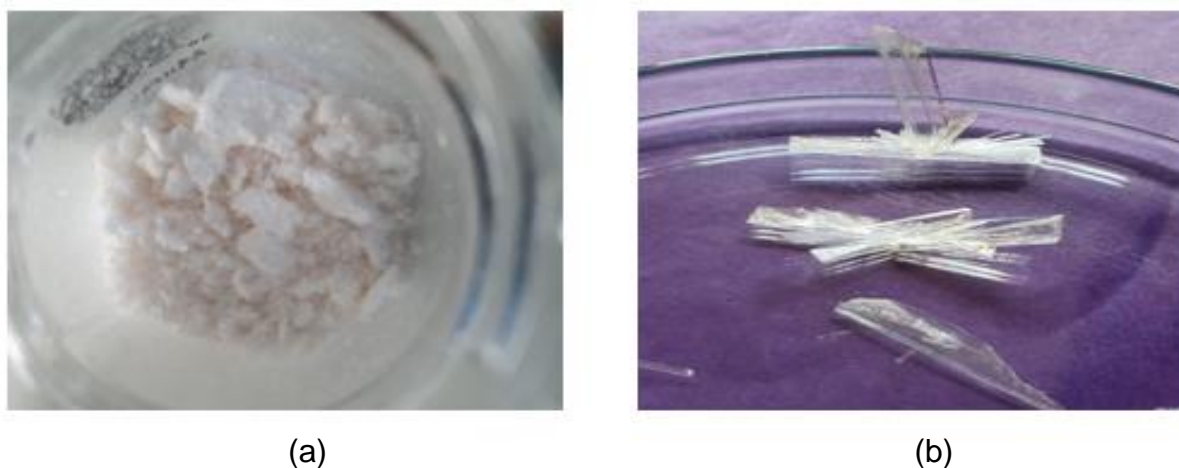
Figura 1. Compuesto alil 4-hidroxifenilcarbamato (A4HPHC). a) Sólido cristalino del A4HPHC obtenido por precipitación en hexano. a) Cristales del A4HPHC obtenidos por recrystalización.
