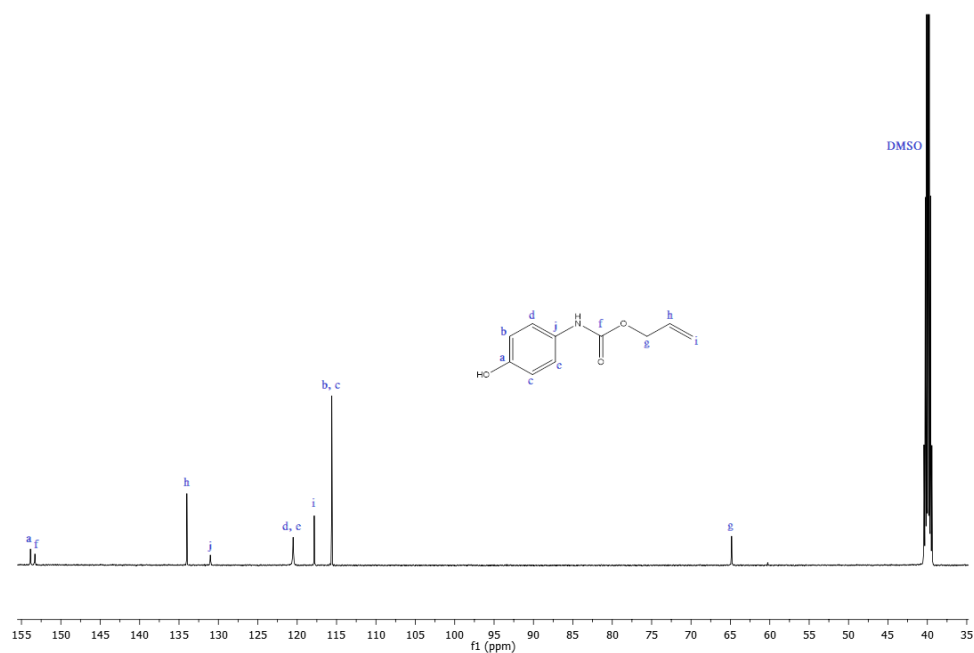
Figura 4. Espectro de RMN 13 C, (500 MHz, DMSO) del A4HPc.
