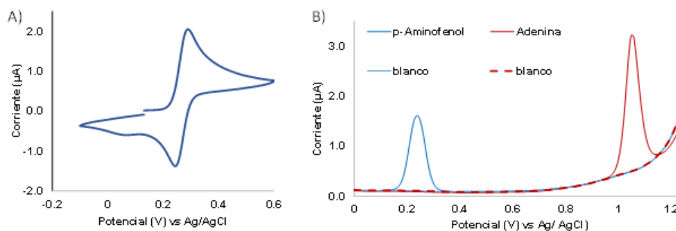
Figura 2. A) VC de PAP [2.5 µg/mL] a 100mV/s, en SAA, 0.1 M, pH 4.5, electrodo pasta de carbón. B). VDP's de p-aminofenol y adenina a una concentración 2.5 g/mL, en SAA pH 4.5. Electrodo pasta de carbono.
