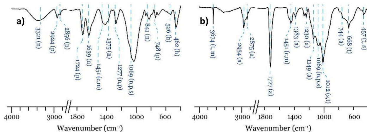
Figura 3. Espectros FTIR-ATR de a) capa frontal negra y b) capa intermedia amarilla. Se indican las señales de nitrocelulosa (n), resinas alquídicas y ftalatos (p), acrílico (a), \text{CaCO}_3 (c), \text{MgCO}_3 (m), óxidos de silicio (s), hematita (h) y talco (t).
