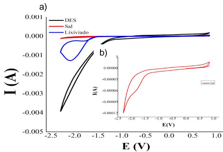
Figura 1. Comparación de voltamperometría del DES- Reline (-), sal de \text{AlCl}_3 (-) y el lixiviado generado del tetra pak (-).
