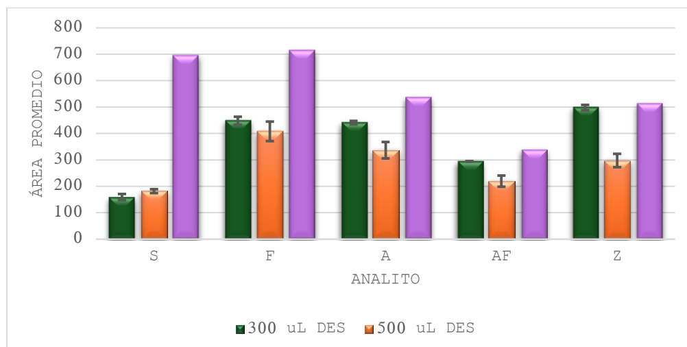
Figura 3. Comparación de la extracción utilizando 300 y 500 \mu\text{L} del DES AD-Mentol (2:1)
