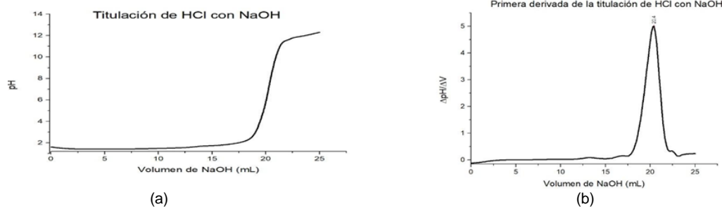
Figura 2. Gráficos obtenidos en la titulación de HCl con NaOH por potenciometría. a) Curva pH-métrica: \text{pH} = f(V) . b) Curva de la primera derivada del pH con respecto al volumen.
