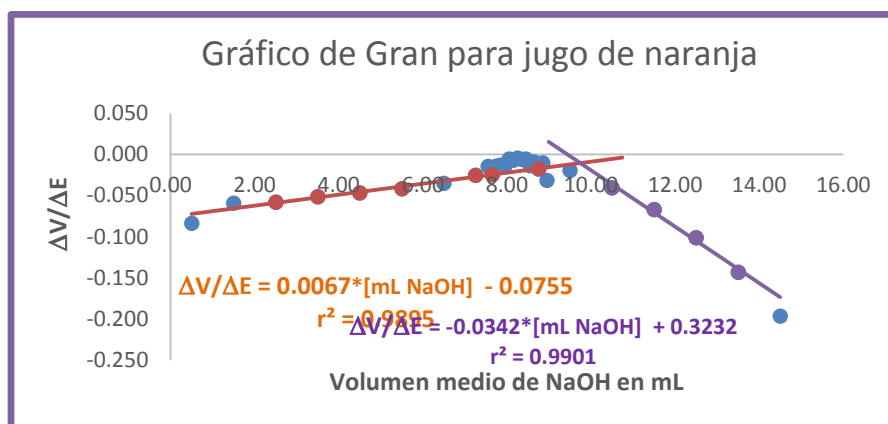
Figura 5. Gráfico de Gran para jugo de naranja
