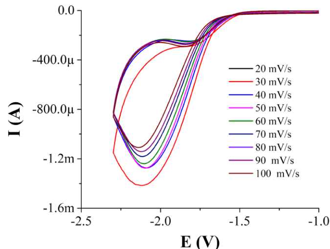
Figura 2. Estudio de velocidad de voltamperometría cíclica del lixiviado con Reline del tetra pak para la electrorecuperación del Aluminio.
