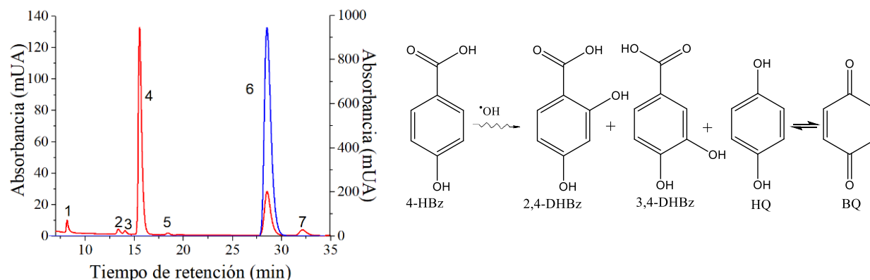
Figura 1. Cromatograma de los productos de descomposición de una solución 0.25 \text{ mmol/dm}^3 del ácido 4-HBz en ambiente airado e irradiado a 10.7 \text{ kGy} (rojo y absorbancia a la izquierda), en azul muestra sin irradiar (absorbancia a la derecha). Los picos corresponden a los siguientes productos: 1) 3,4,5-THBz, 2) BQ, 3) 2,3,4-THBz, 4) 3,4-DHBz, 5) Cat, 6) 4-HBz y 7) 2,4-DHBz. Reacción de oxidación del ácido 4-HBz de una solución saturada con N_2O y sus productos radiolíticos primarios.
