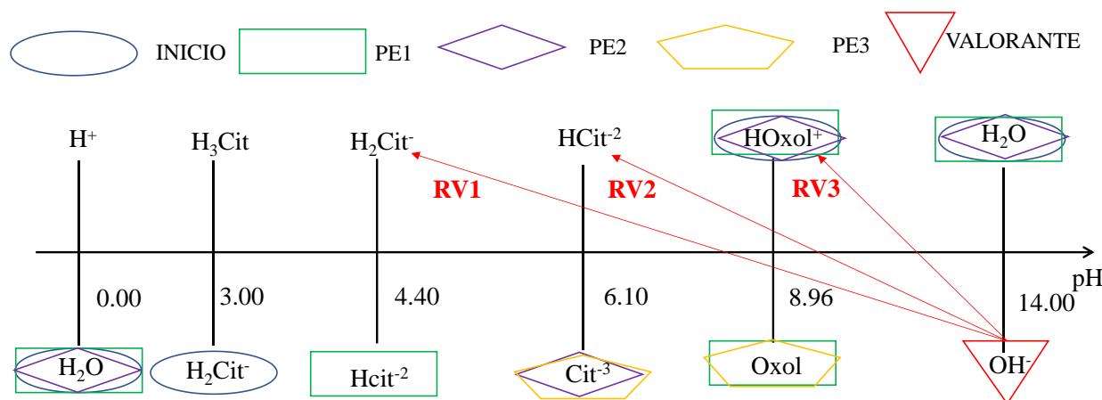
Figura 2. Resumen de las EPRx de la valoración de un volumen de solución de citrato de oxalamina con hidróxido de sodio.
