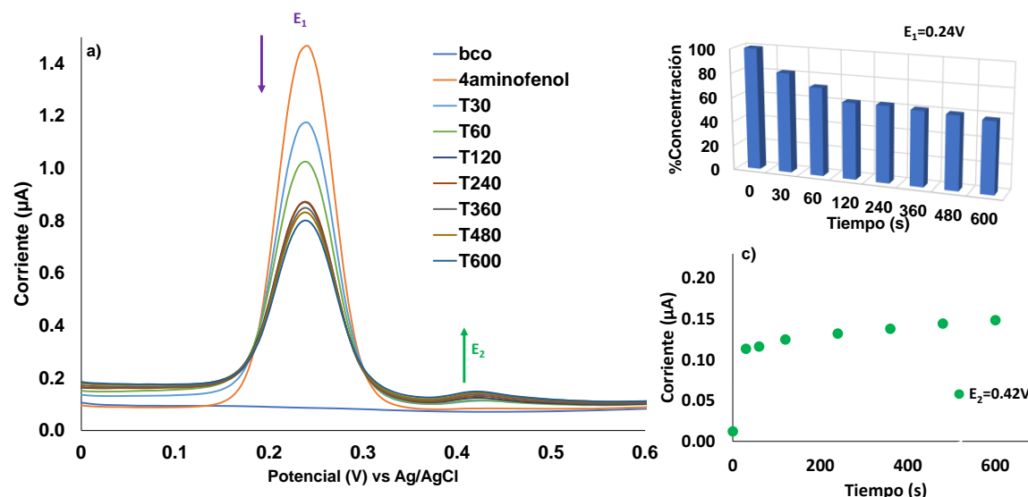
Figura 4. a) DPV's oxidación de PAP E_a = 0.3 durante 30, 60, 120, 360, 240, 480, 600 y 700 s, en SAA pH 4.5. Electrodo pasta de carbono. b) gráfico de % de concentración remanente de PAP después del estrés oxidativo. c) Gráfico del incremento de la corriente correspondiente a la especie oxidada del PAP vs tiempo.
