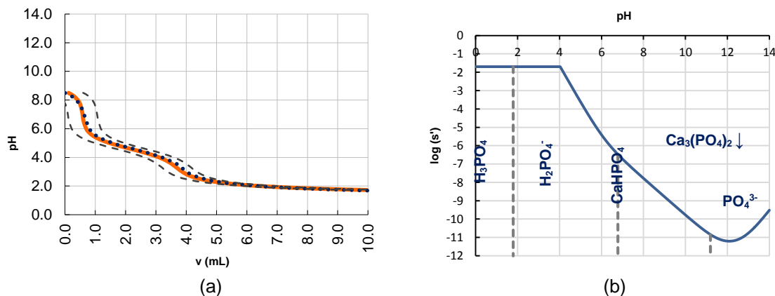
Figura 4. Control del buffer de Britton-Robinson mediante la adición de \text{Ca}^{2+} como agente enmascarante de fosfato. a) Ajuste no lineal típico de la curva de titulación del buffer tras el retiro de fosfatos insolubles. b) Diagrama de \log(s') = f(\text{pH}) de las especies de fosfato (0.02 mol/L) a \text{pCa}' = 1.48 .
