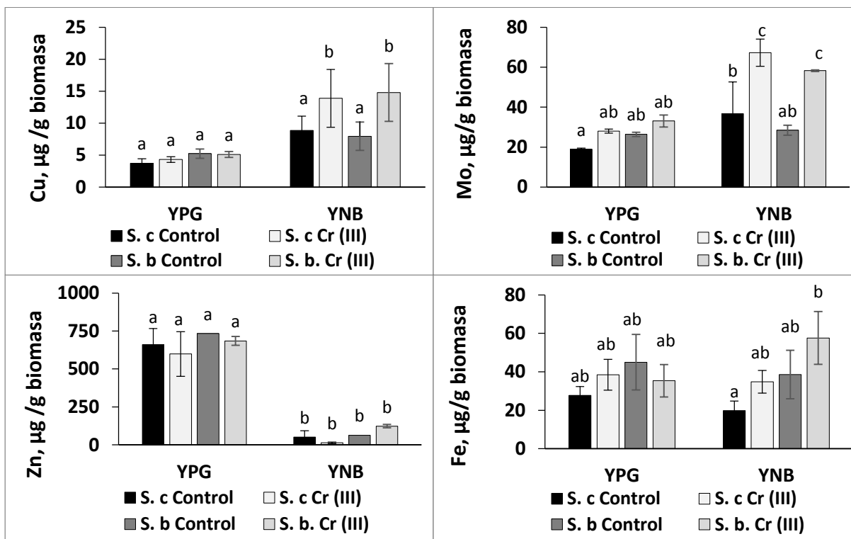
Figura 2. Perfil de elementos minoritarios (Cu, Mo, Zn y Fe) obtenidos de la biomasa digerida con \text{HNO}_3 y determinadas por MP-AES. La biomasa se obtuvo de células de levaduras cultivadas en medio YPG y YNB en presencia y ausencia de Cr (III). Los resultados son expresados en cantidad ( \mu\text{g} para Cu, Mo, Fe y Zn) del elemento por g de biomasa. Las letras distintas sobre las barras indican diferencias significativas entre las medias según la prueba Tukey para p \geq 0.5 .
