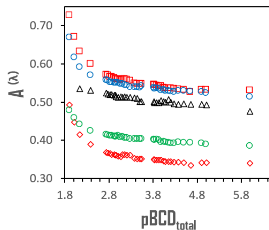
Figura 3. Valores de absorción, A , como una función del p\beta\text{CD}_{\text{total}} a diferentes longitudes de onda para cada valor de pH. pH = (1.22 \pm 0.01) : \square A^{(272)} , \diamond A^{(248)} ; pH = (6.55 \pm 0.01) : \circ A^{(245)} , \circ A^{(274)} ; pH = (13.38 \pm 0.01) : \Delta A^{(274)} .
