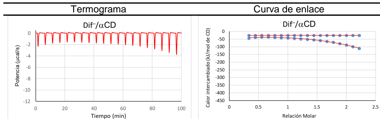
Figura 4. Termogramas y curvas de enlace para la interacción de Dif - con las CDs. Las curvas superiores en las gráficas de la derecha corresponden al calor de dilución.
