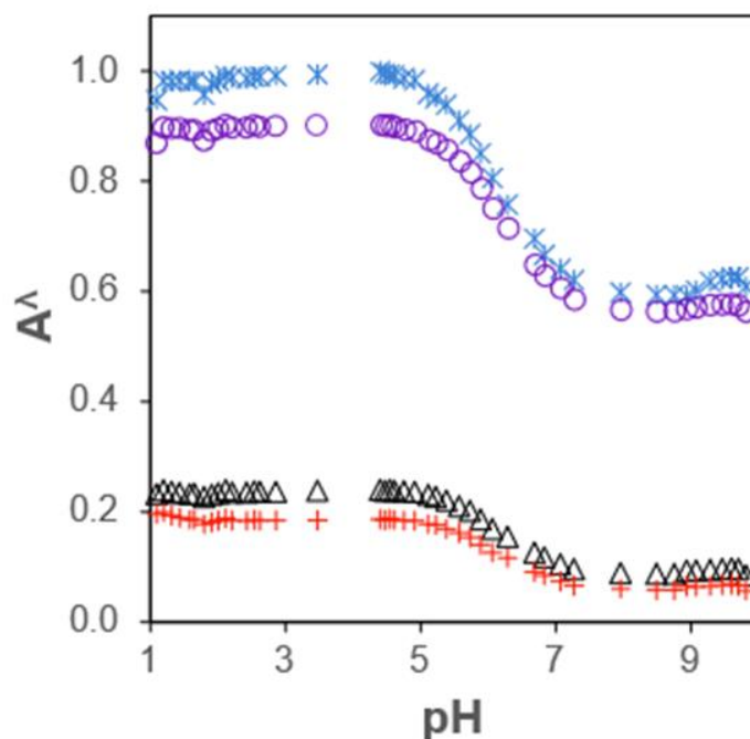
Figura 3. Valores de absorbancia, A_\lambda , como una función del pH a diferentes longitudes de onda. (X) \lambda = 208 nm, (o) \lambda = 281 nm, ( \Delta ) \lambda = 306 nm y (+) \lambda = 319 nm.
