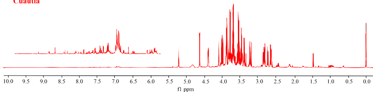
Figura 1. Espectros ^1\text{H} -RMN a 750 MHz representativos de tres cultivares de verdolaga ( Portulaca oleracea L.) en función de la dosis de nitrógeno en hidroponía en el intervalo de \delta -0.5 a 10.0 ppm, y las expansiones para el rango de \delta 6.5 a 9.0 ppm. Cultivares (A) Xochimilco, (B) Mixquic, y (C) Cuautla.
