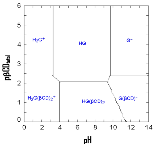
Figura 5. Diagrama de zonas de predominio construido con las constantes de formación calculadas en este trabajo para el sistema \beta -ciclodextrina/guanina a través de la herramienta computacional MEDUSA.
