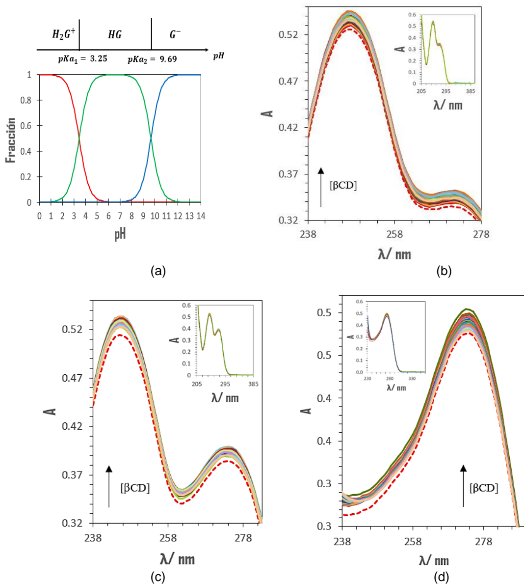
Figura 2. a) Diagrama de distribución de la guanina en medio acuoso. b) Espectros de UV de la guanina 70.44 \mu M a pH = (1.22 \pm 0.01) para diferentes concentraciones de \beta CD. c) Espectros de UV de la guanina 70.44 \mu M a pH = (6.55 \pm 0.01) para diferentes concentraciones de \beta CD. d) Espectros de UV de la guanina 70.44 \mu M a pH = (13.38 \pm 0.01) para diferentes concentraciones de \beta CD. La línea punteada roja en los incisos b, c y d son los espectros de la guanina en ausencia de \beta CD.
