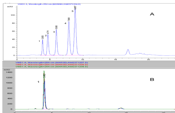
Figura 1. Cromatogramas obtenidos para: A) Una solución estándar de parabeno a una concentración de 2 mg/mL y B) Muestra 1 (enjuague bucal) ambos empleando el método de MIL´s-DLLME y cromatografía descritos. 1. Metilparabeno, 2. Etilparabeno, 3. Propilparabeno, 4. Butilparabeno, 5. Bencilparabeno.
